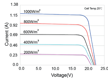
Curvas I-V del módulo PV ESF-20PA I-V Curves of PV module ESF-20PA
