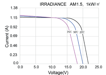
Curvas I-V del módulo PV ESF-20PA a varias temperaturas de célula I-V Curves of PV module ESF-20PA at various cell temperatures
