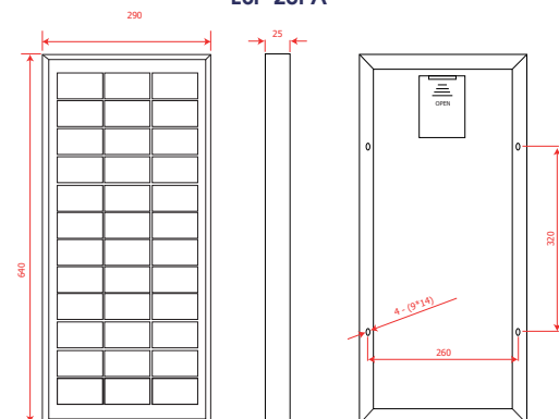
Dimensiones - Dimensions ESF-20PA
