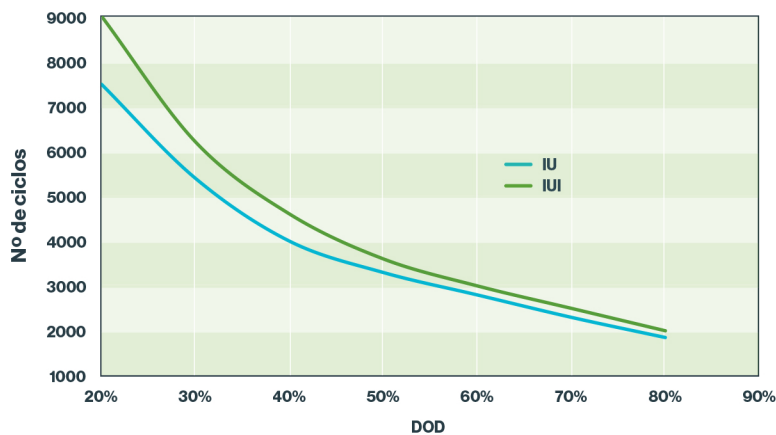
OPzS Solar - Ciclos vs DOD & 20°C
